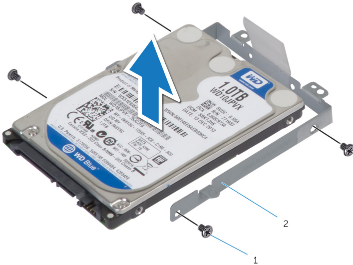
1 (ברגים) 2 תושבת הכונן הקשיח
