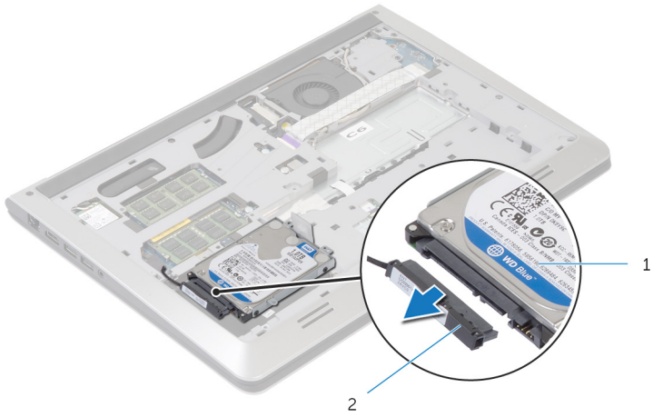
1 מכלול כונן קשיח 2 כבל הכונן הקשיח
