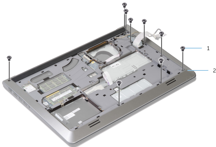
1 ברגים (9) 2 מסגרת הבסיס
